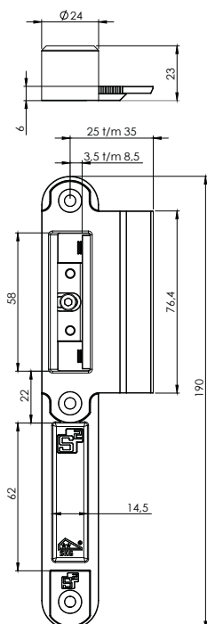
Flexi hoofsluitkom korte lip
