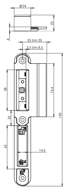
Flexi hoofdsluitkom korte lip
